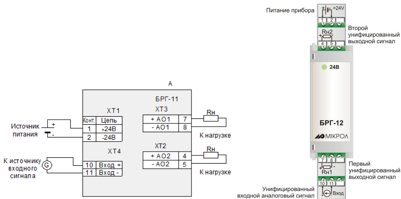
Рисунок 3.3 - Схема электрических подключений преобразователя БРГ-12
